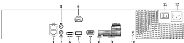
DS-7732NI-I4
