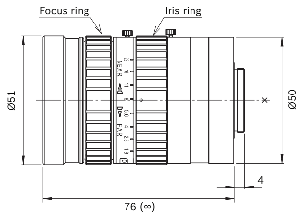
Dimensions LFF-8012C-D75
