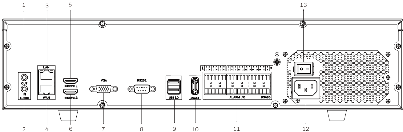
HN353208xxNR/HN356408xxNR
