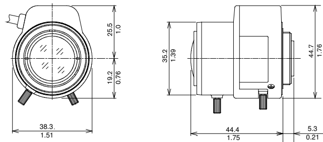
Dimensions LTC 3664/30
